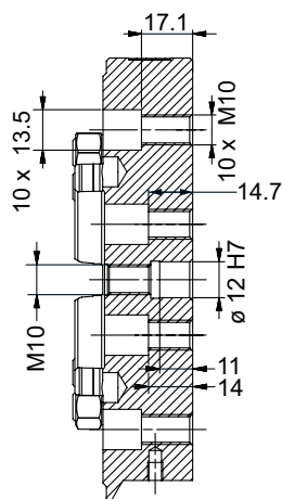
Schnitt A - A
